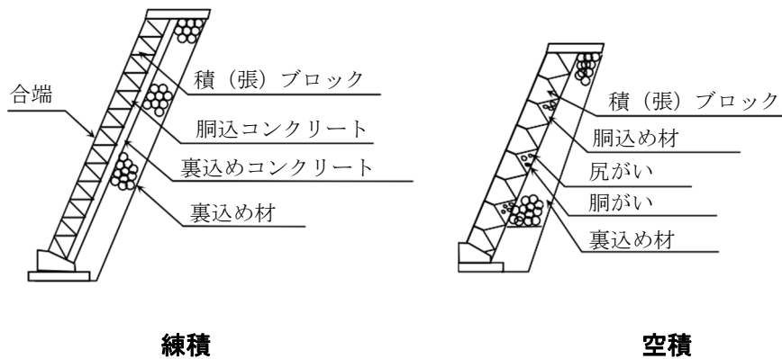
図 3-3-4 コンクリートブロック工
