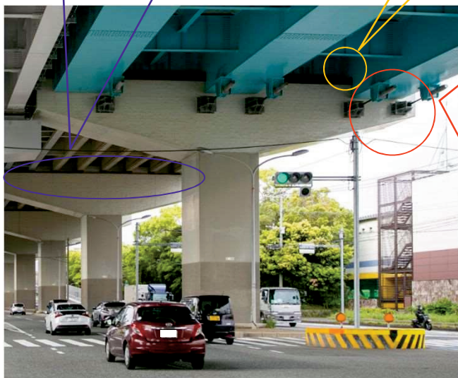
橋脚の桁かかり部分を拡幅
